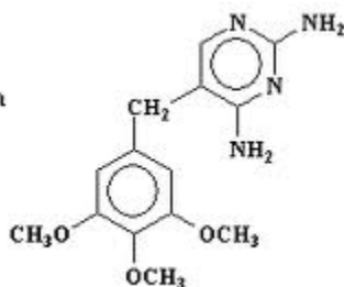
Trimethoprim C_{14}H_{18}N_4O_3
